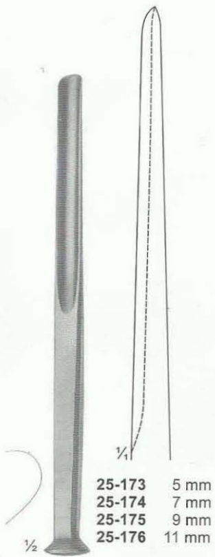
ALEXANDER 25-173 - 176 Gouges 170 mm
