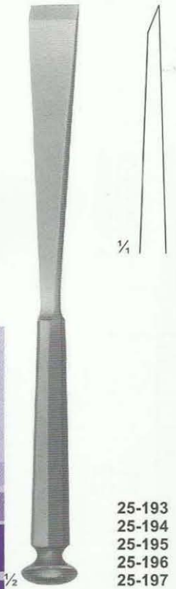
STILLE 25-193 - 197 Chisels 205 mm
